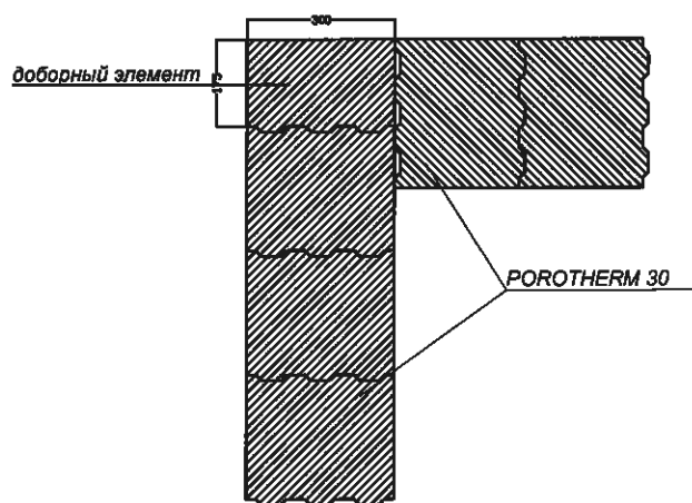
Четный ряд кладки
