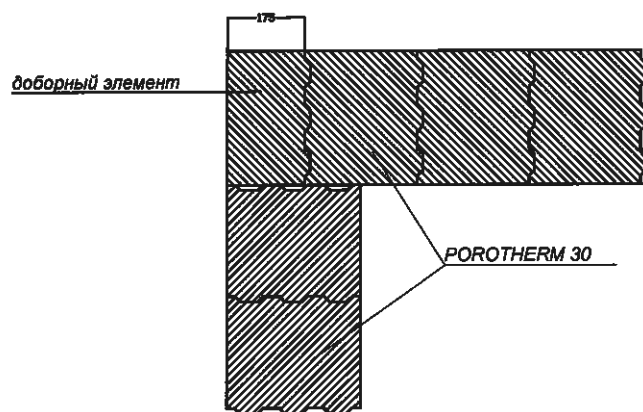
Нечетный ряд кладки
