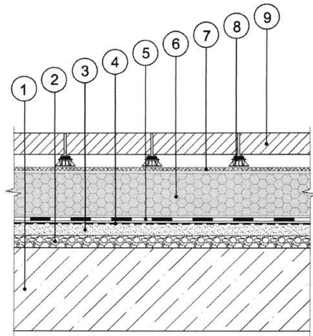
Рис. 10. Кровельная система № 10
