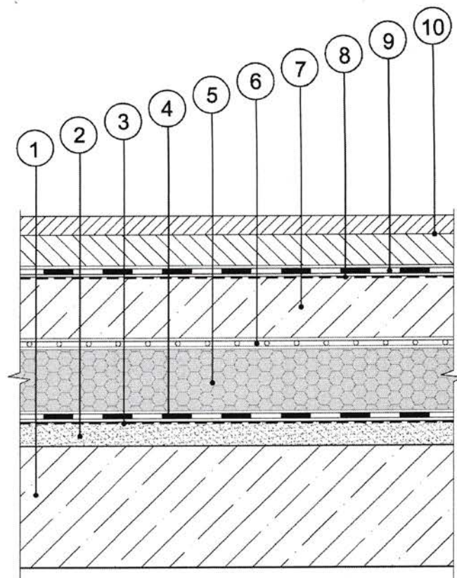
Рис. 7. Кровельная система № 7
